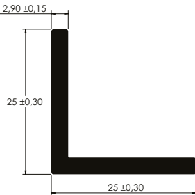
ÁNGULO DE 1" 1" Angle
