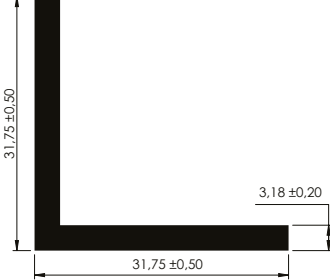
ÁNGULO DE 1-1/4" 1-1/4" Angle
