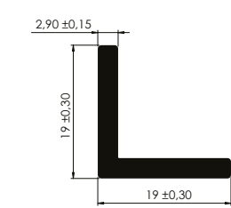
ÁNGULO DE 3/4" 3/4" Angle
