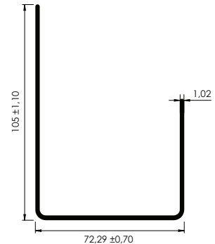
EMPALME DE CANAL Gutter Splice
