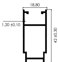
TRASLAPE REFORZADO Stile Reinforced
