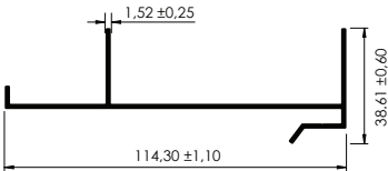
BORDE DE GOTEO DE 3" 3" Drip Edge Fascia
