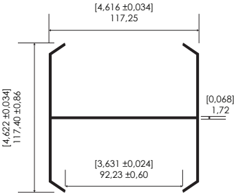
POSTE INTERNO PARA CERCA Post Stiffener
