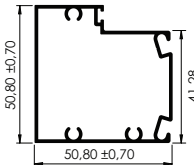
JAMBA DE PUERTA DE 2" x 2" 2" x 2" Door Jamb
