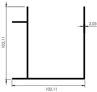
POSTE ESQUINERO Corner Post
