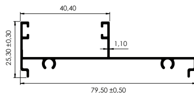
JAMBA Jamb
