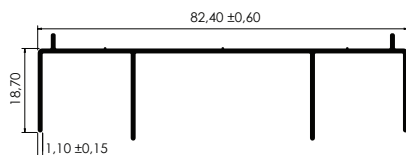
CABEZAL Head
