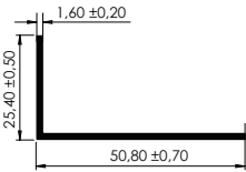
ANGULO 2" x 1" Angle 2"x 1"
