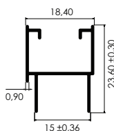
TRASLAPE Stile
