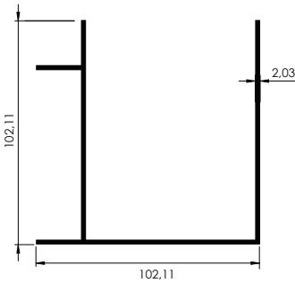
POSTE ESQUINERO Corner Post
