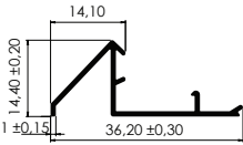
PISAVIDRIO HEMBRA Glass Holder (Female)
