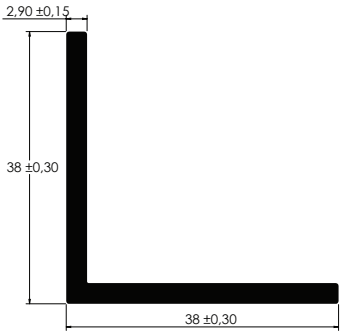
ÁNGULO DE 1-1/2" 1-1/2" Angle
