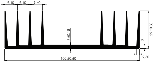
DISIPADOR DE CALOR Heat Sink
