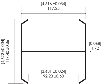
POSTE INTERNO PARA CERCA Post Stiffner
