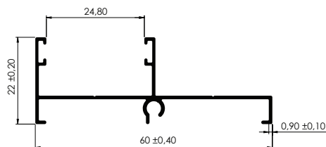
JAMBA Jamb
